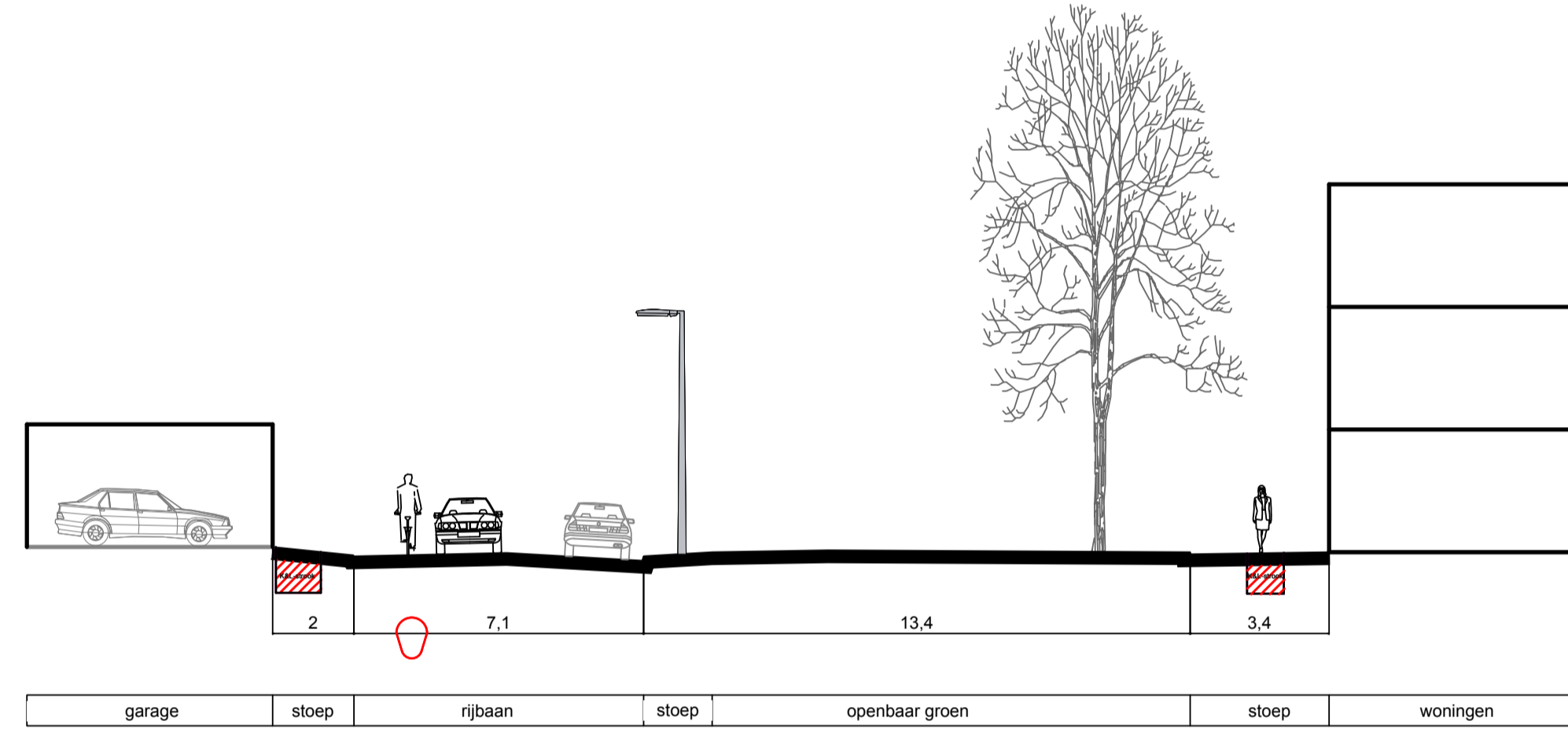
19. Schubertlaan b huidige situatie
