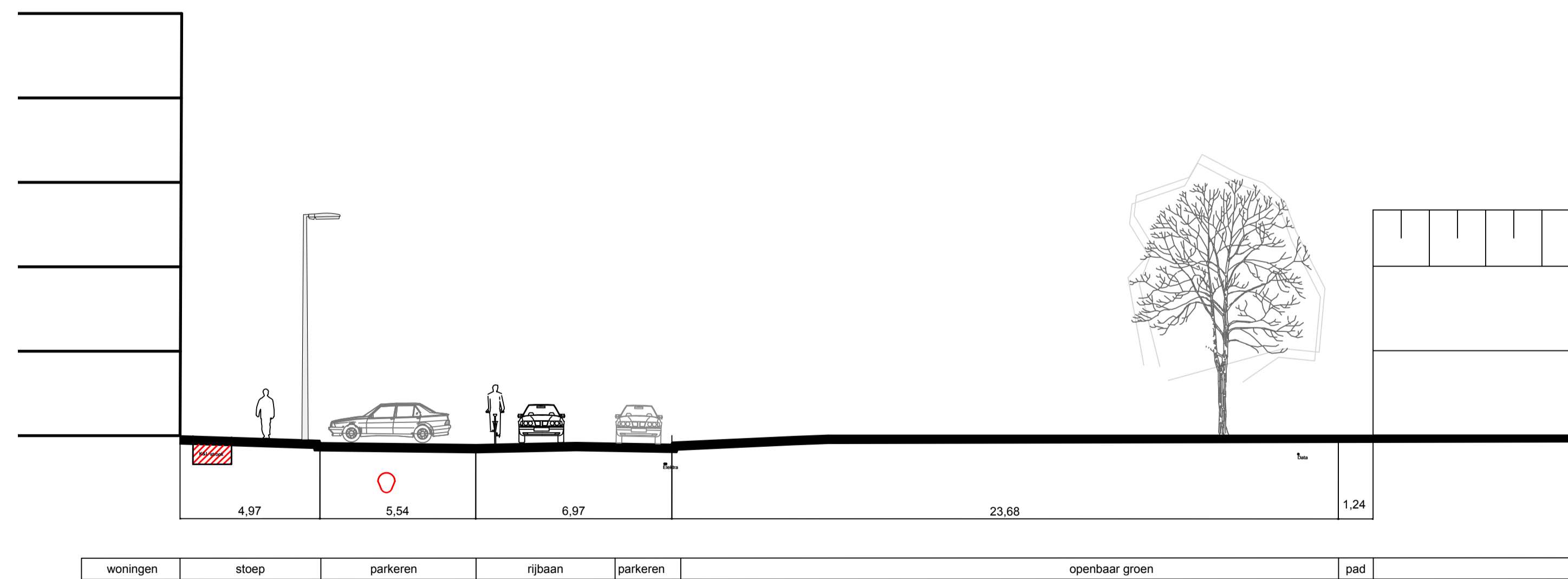
21. Mahlerstraat a huidige situatie
