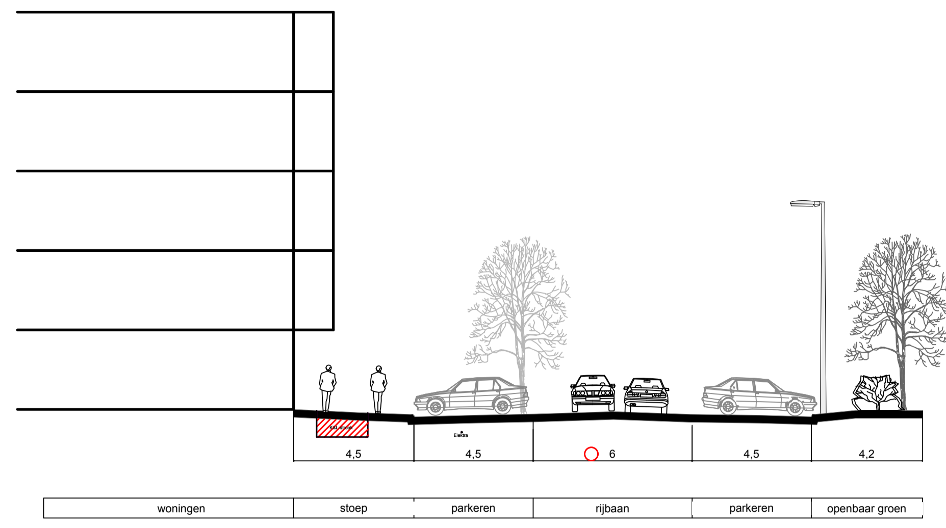
17. Pergolesiepad huidige situatie
