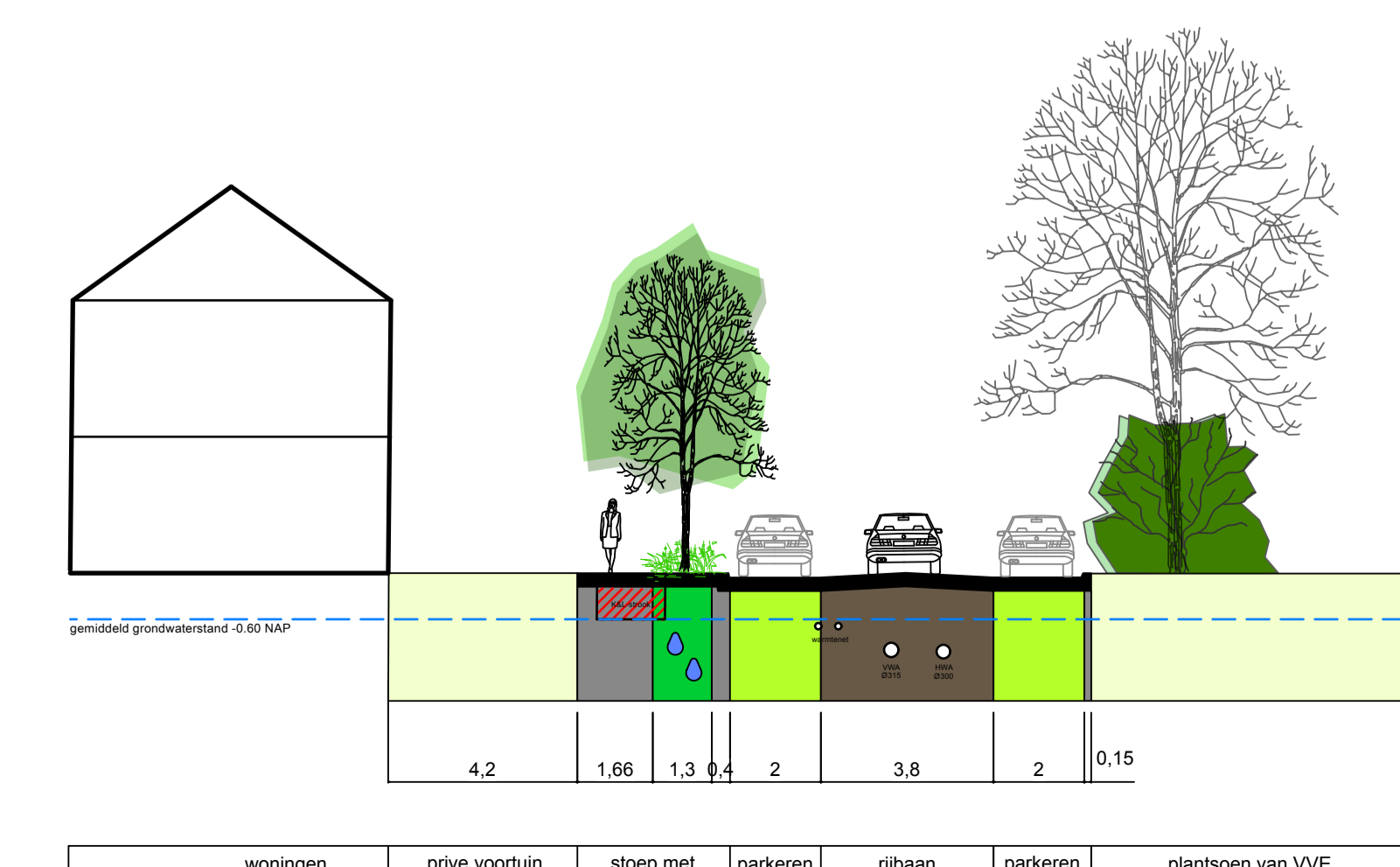
22. Mahlerstraat b toekomstige situatie
