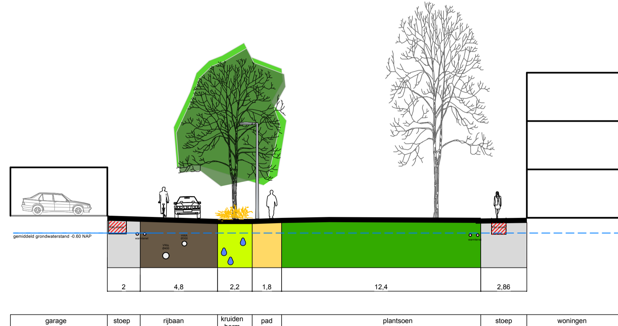
19. Schubertlaan b toekomstige situatie
