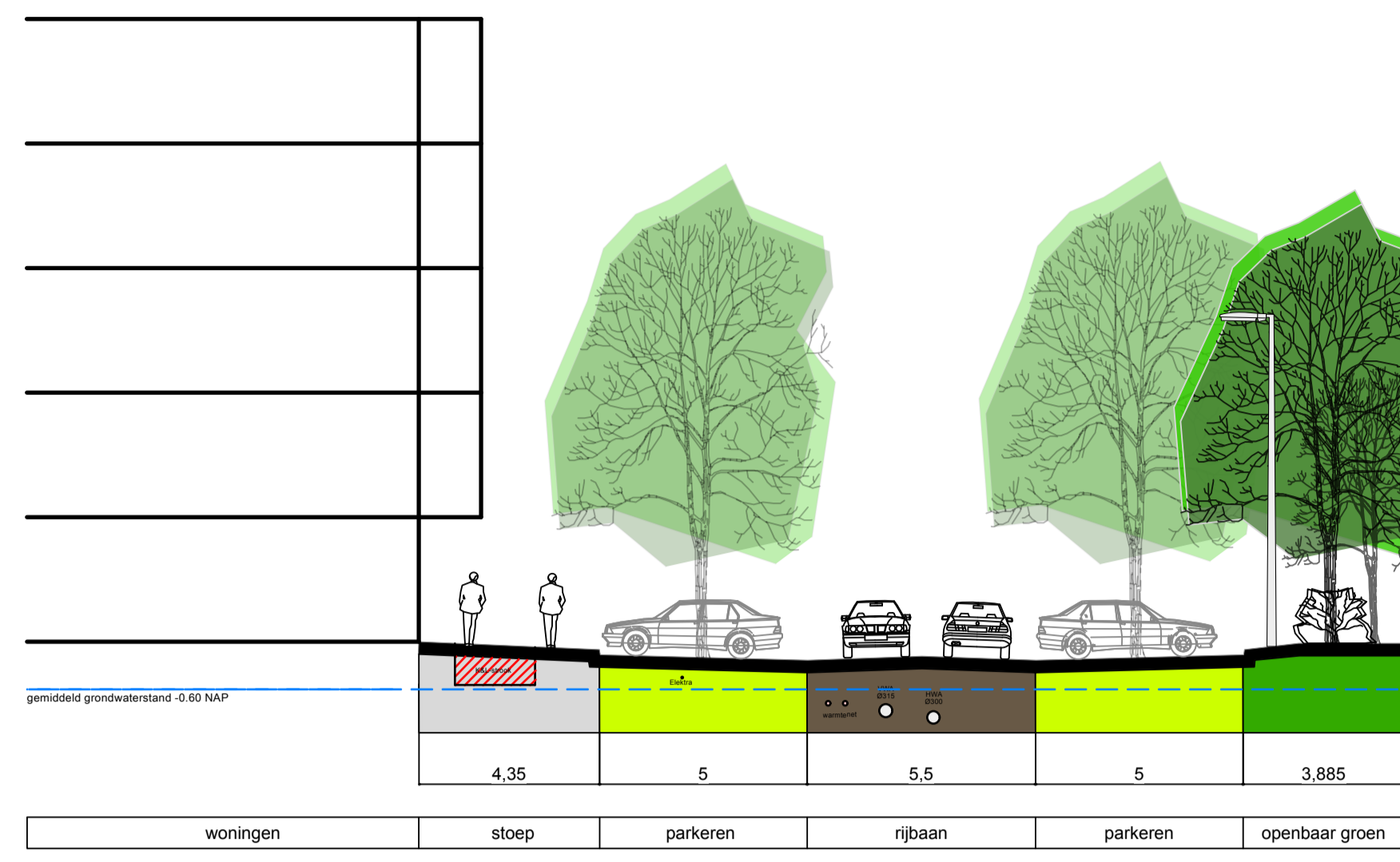
17. Pergolesiepad toekomstige situatie
