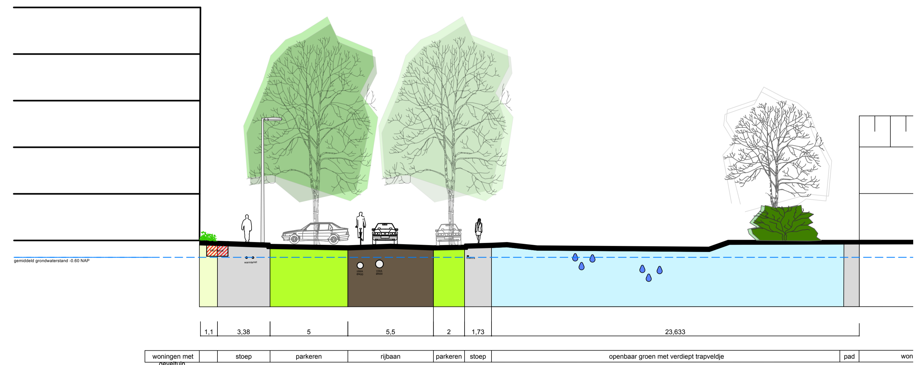
21. Mahlerstraat a toekomstige situatie
