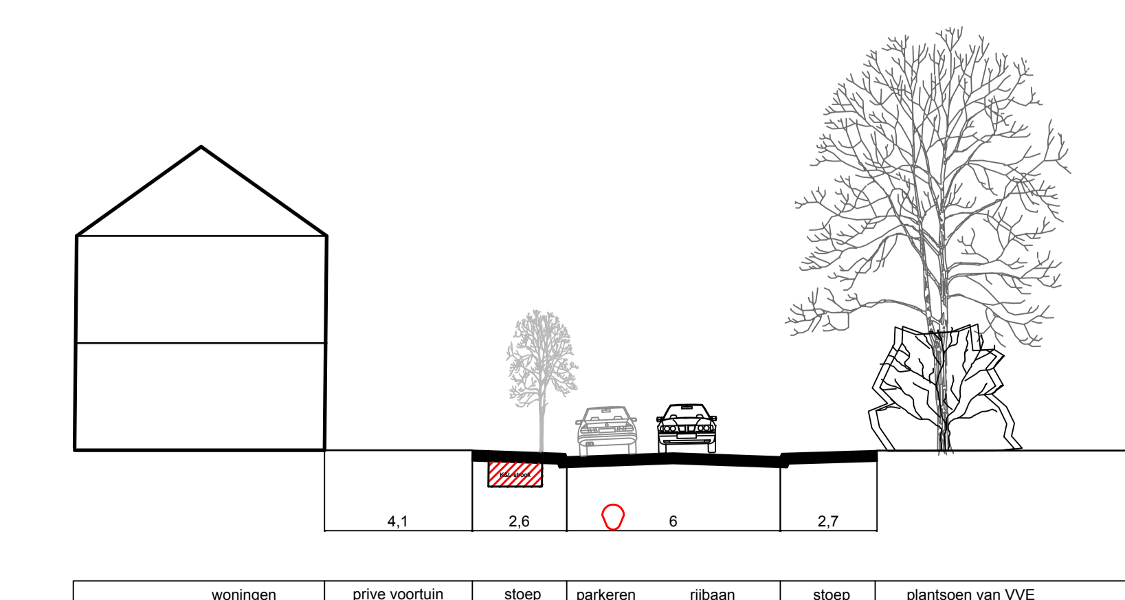
22. Mahlerstraat b huidige situatie
