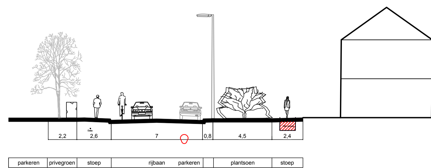
18. Schubertlaan a huidige situatie
