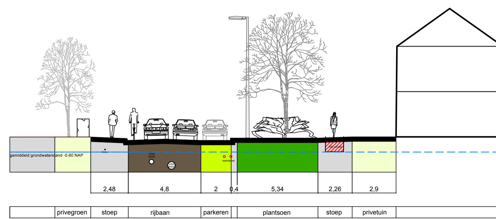
19. Schubertlaan b toekomstige situatie
