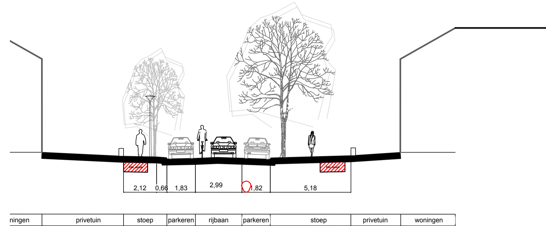
20. Händelstraat huidige situatie
