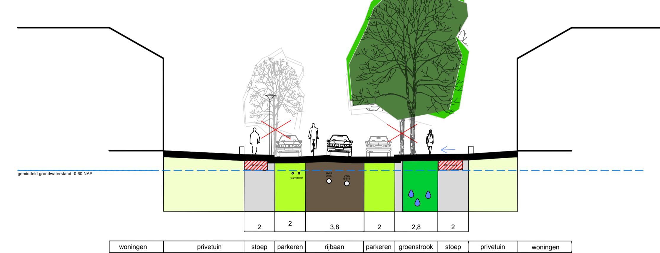
21. Mahlerstraat a toekomstige situatie
