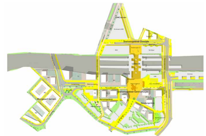
Stedenbouwkundig Plan Stationsgebied Leiden (2012)
