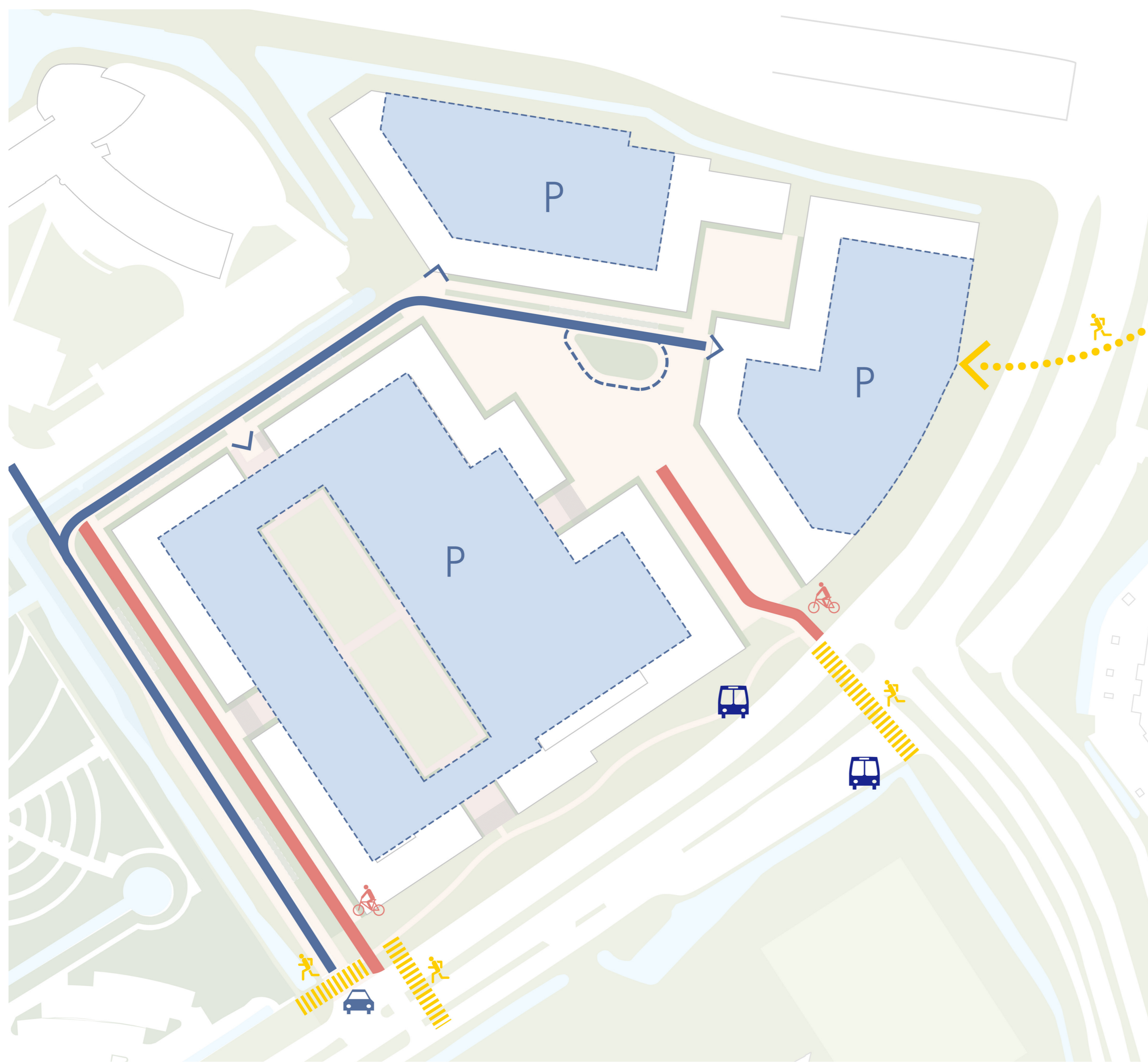
Ontsluitingsprincipe
