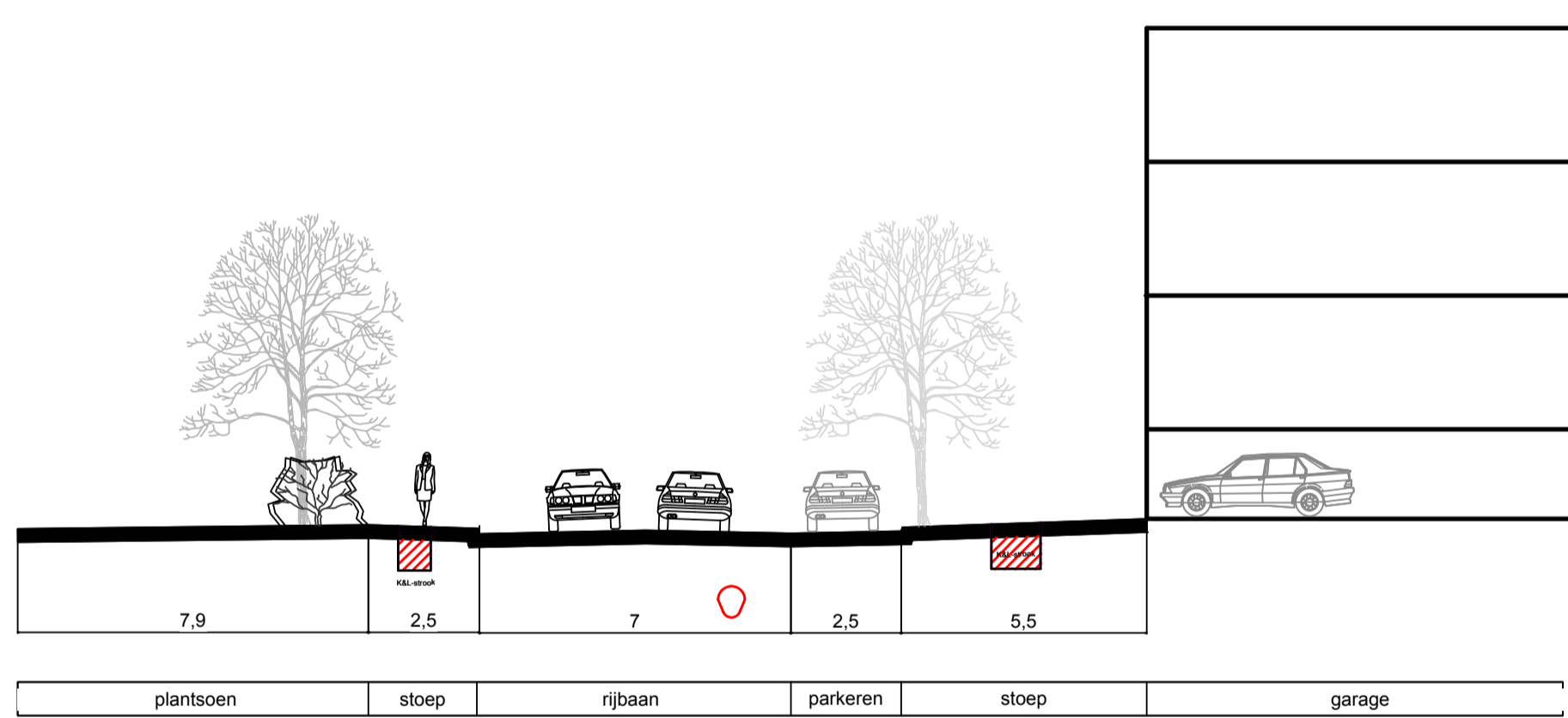
08. Vivaldistraat a huidige situatie
