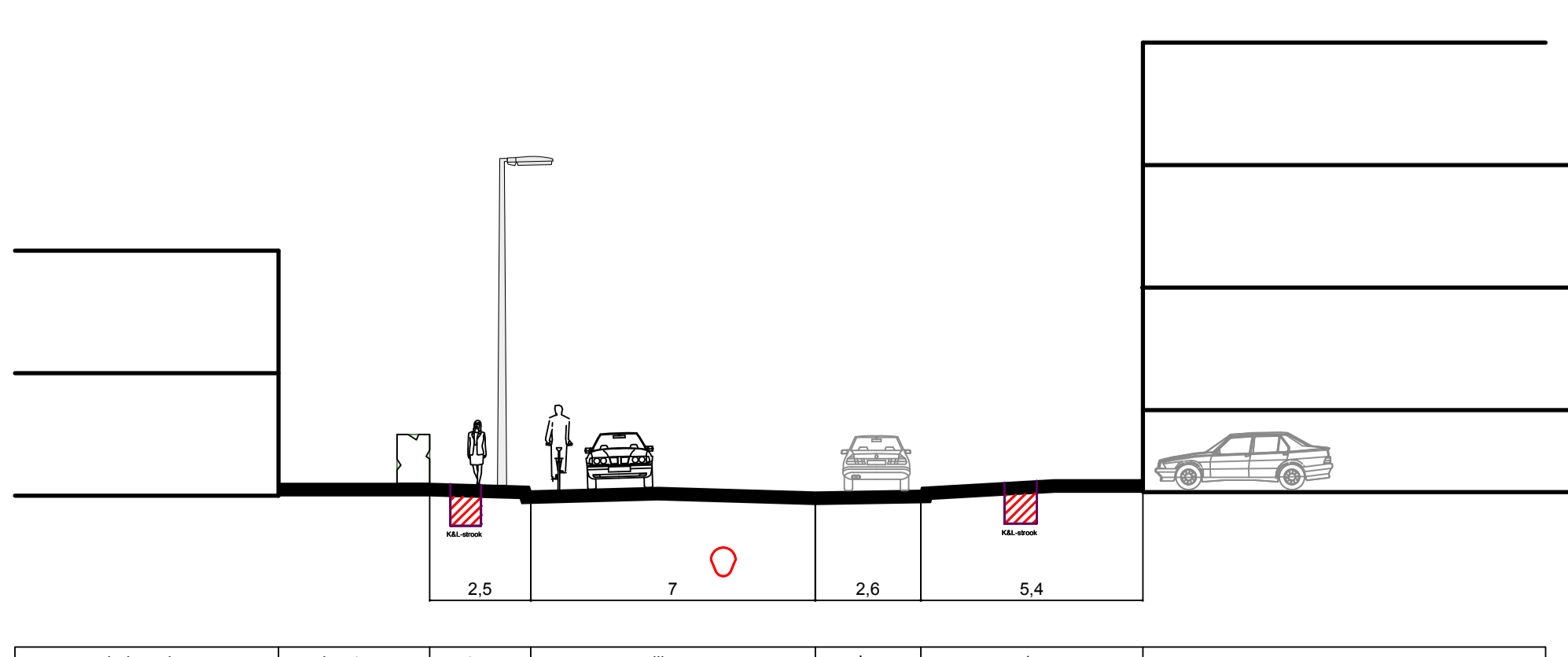
10. Corellistraat a huidige situatie
