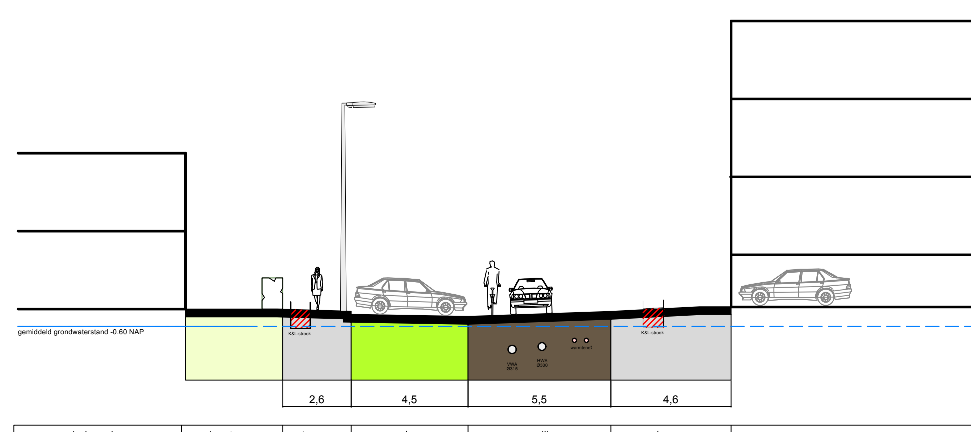
10. Corellistraat a toekomstige situatie
