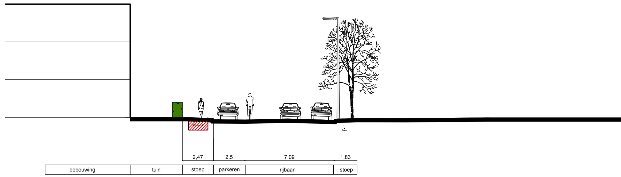
07. Beethovenlaan huidige situatie
