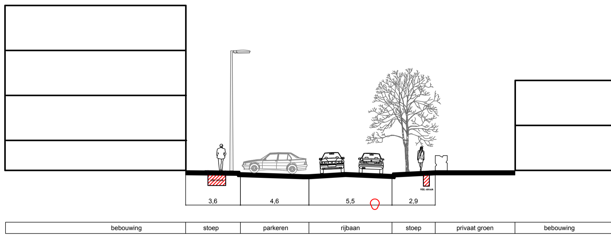
08. Vivaldistraat a huidige situatie
