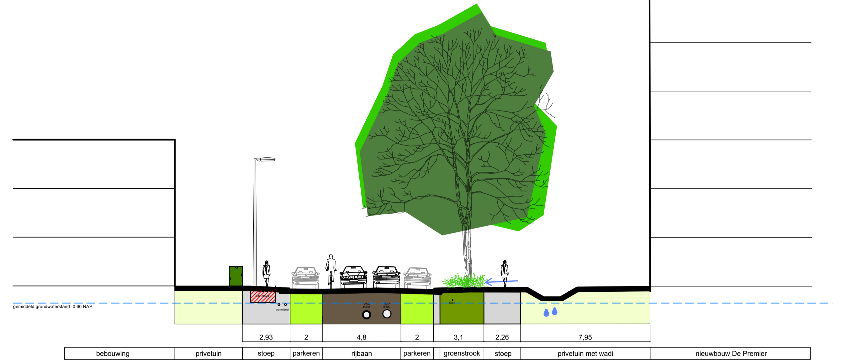
07. Beethovenlaan toekomstige situatie
