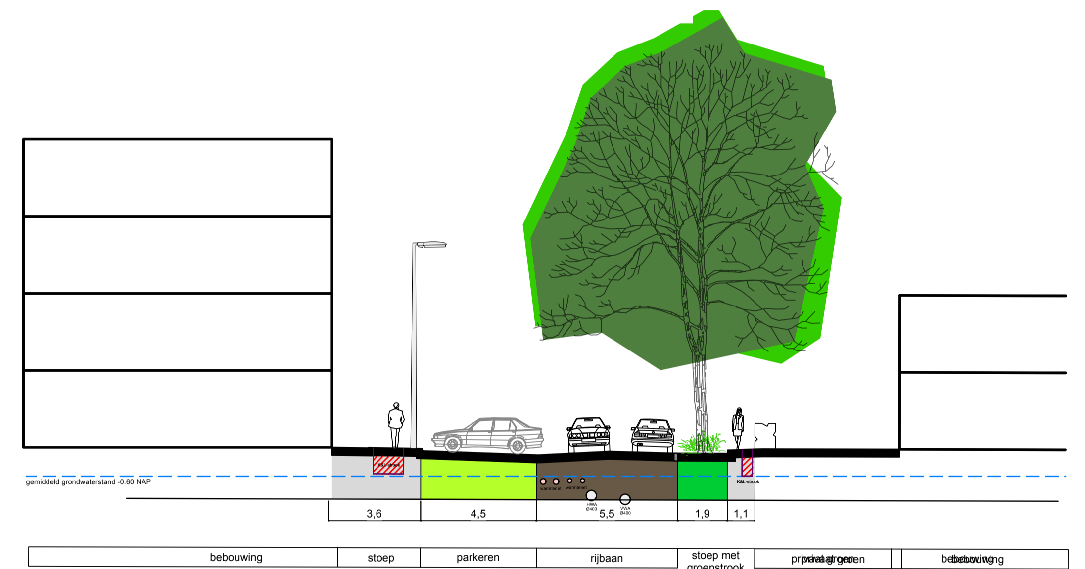
07. Beethovenlaan toekomstige situatie
