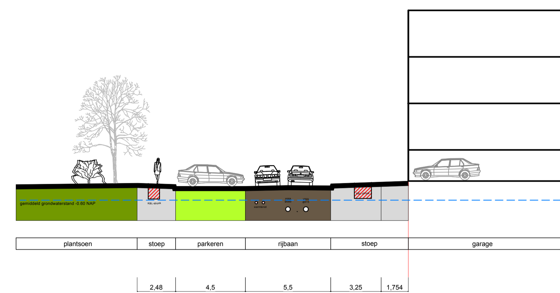
09. Vivaldistraat b toekomstige situatie
